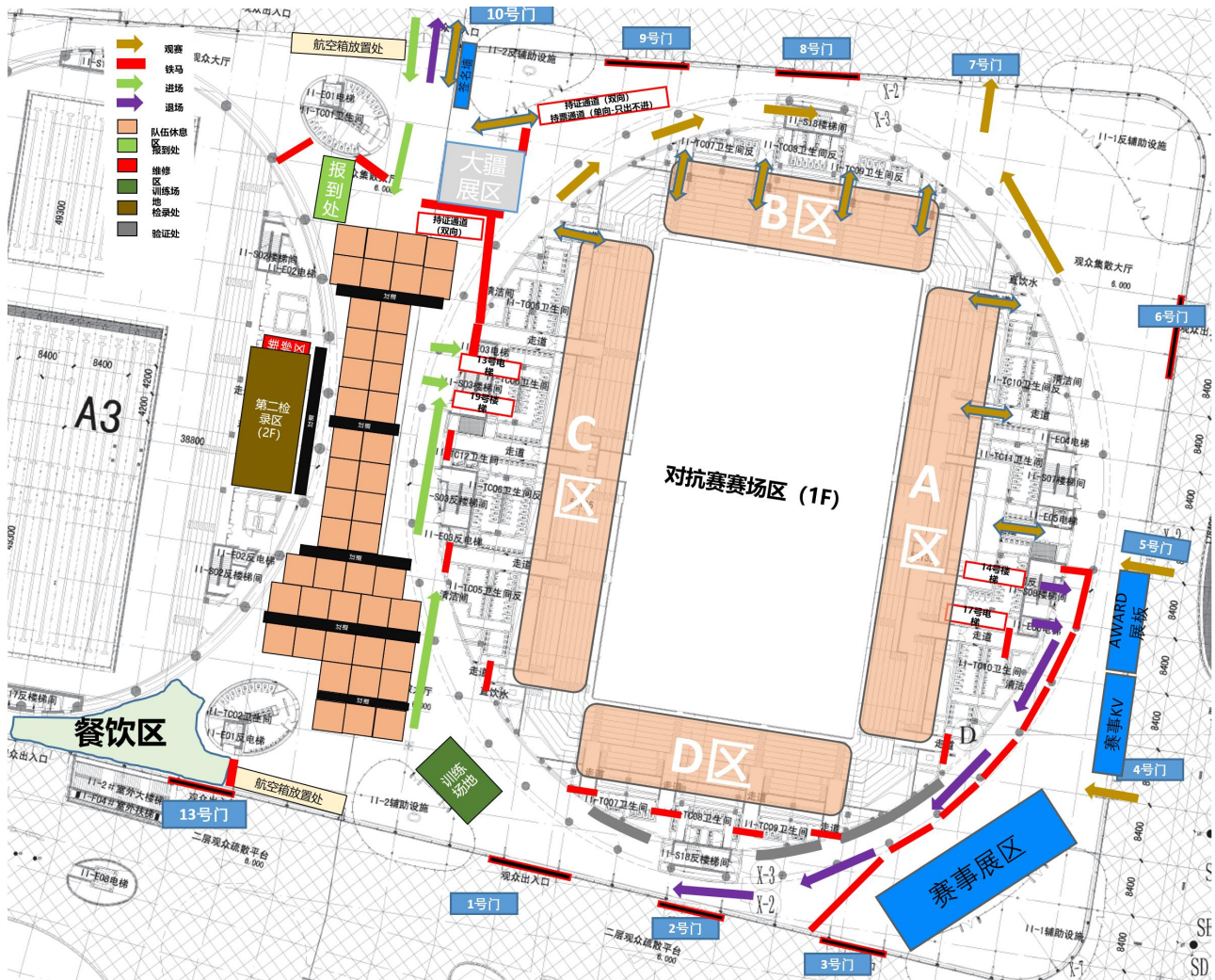
图 4-3 场地规划示意图 - 备场/检录/道具训练区域规划图
